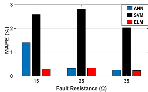
شکل (۱۰): نمودار درصد میانگین خطا بر حسب مقاومت برای مقاومت‌هایی که در فرآیند آموزش استفاده نشده‌اند
