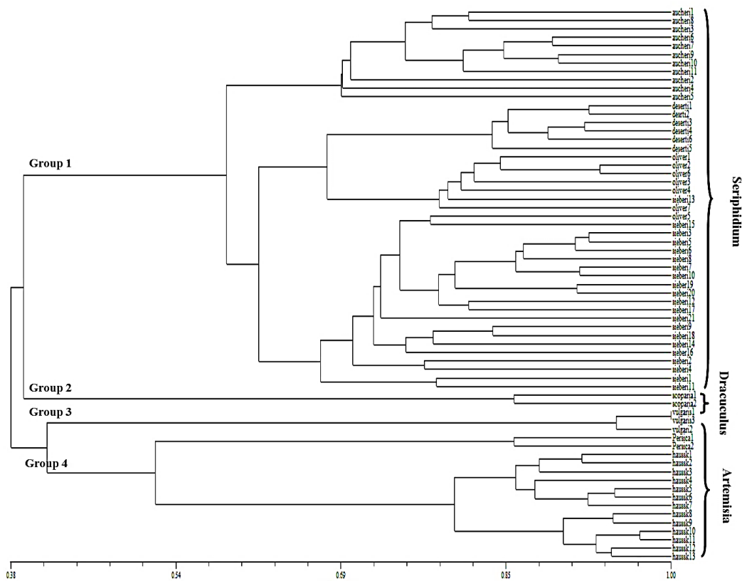
شکل ۴- دندروگرام حاصل از بررسی داده‌های ریخت‌شناسی ۶۴ گونه Artemisia و آنالیز عددی از نرم‌افزار NTsys 2.02
