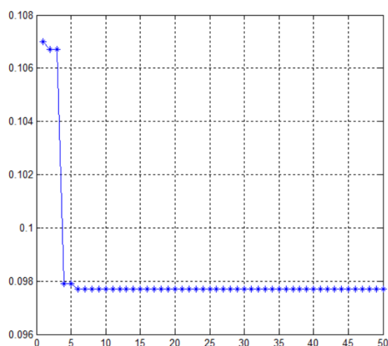
شکل (۱۳): روند همگرایی تابع هدف - سناریو دو با در نظر
