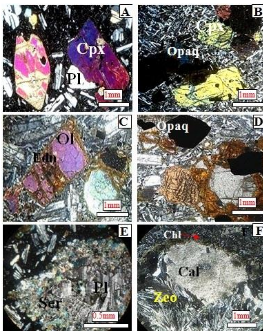
شکل ۳- تصاویرهای میکروسکوپی (در XPL) از منشورهای بازالتی شهرستان گرمی (استان اردبیل): (A) فنوکریست‌های پلاژیوکلاز و کلینوپیروکسن با بافت هیالومیکرولیتی پورفیری؛ (B) بافت گلومروپورفیریتیک پدیدآمده از گردهم‌آمدن کلینوپیروکسن و
