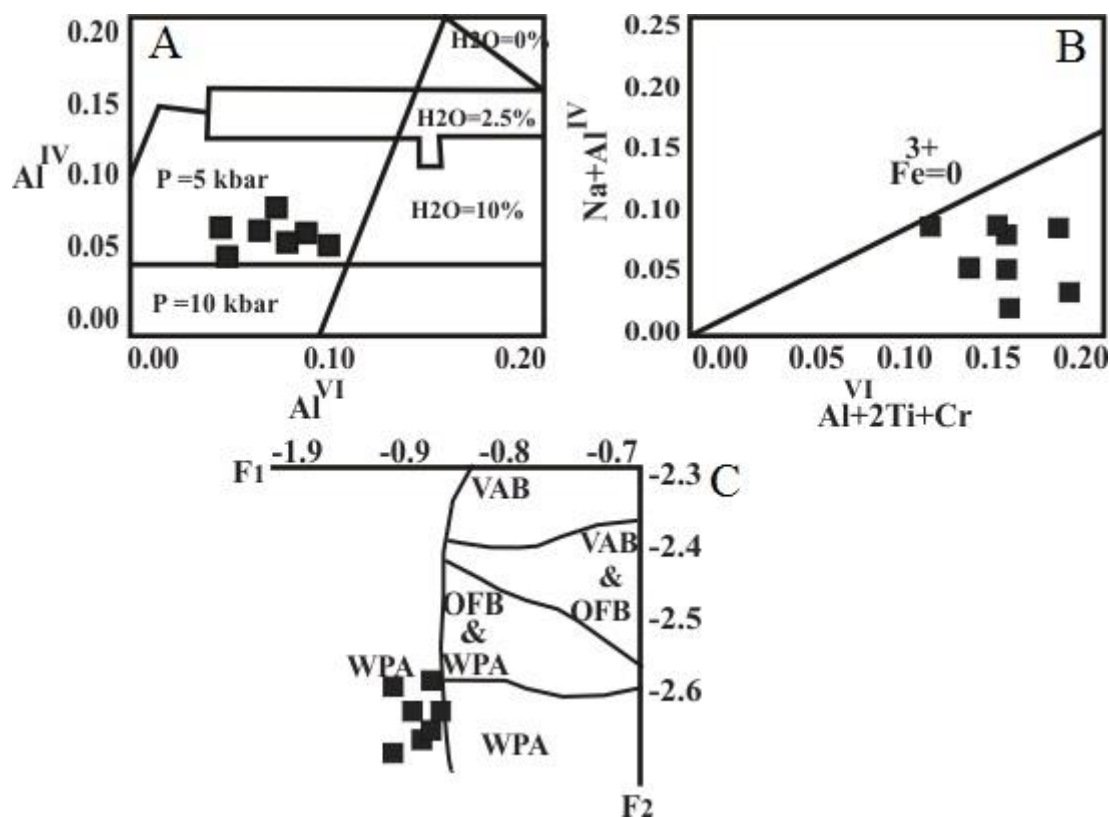
شکل ۵- داده‌های شیمیایی کانی‌های سازنده بازالت‌های منشوری شهرستان گرمی (استان اردبیل) در: (A) نمودار توزیع آلومینیم چهاروجهی (تتراهدری) و هشت‌وجهی (اکتاهدری) در کلینوپیروکسن‌ها (Coltorti et al. , 2007)؛ (B) نمودار تغییرات Al^{VI}+2Ti+Cr در برابر Na+Al^{IV} (Marcelot et al. , 1983)؛ (C) نمودار F_1 در برابر F_2 (Nisbet and Pearce, 1989) برای شناسایی محیط پیدایش کلینوپیروکسن‌ها (WPA: Within plate Alkaline Basalts; WPT: Within plate tholeiitic basalts; (OFB: Ocean- Floor Basalts; VAB: Volcanic Arc Basalts
