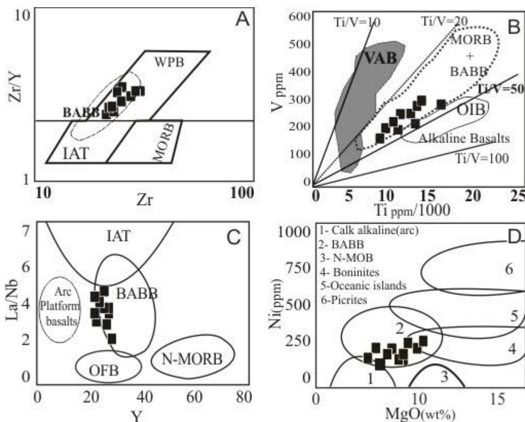
شکل ۹- شناسایی پهنه زمین‌ساختی بازالت‌های منشوری شهرستان گرمی (استان اردبیل) در: (A) نمودار Zr در برابر Zr/Y (Floyd et al. , 1991); (B) نمودار Ti/1000 در برابر V (Pearce and Norry, 1979); (C) نمودار Y در برابر La/Nb (Shervais, 1982); (D) نمودار Ni در برابر MgO (Juteau and Maury, 1999).
