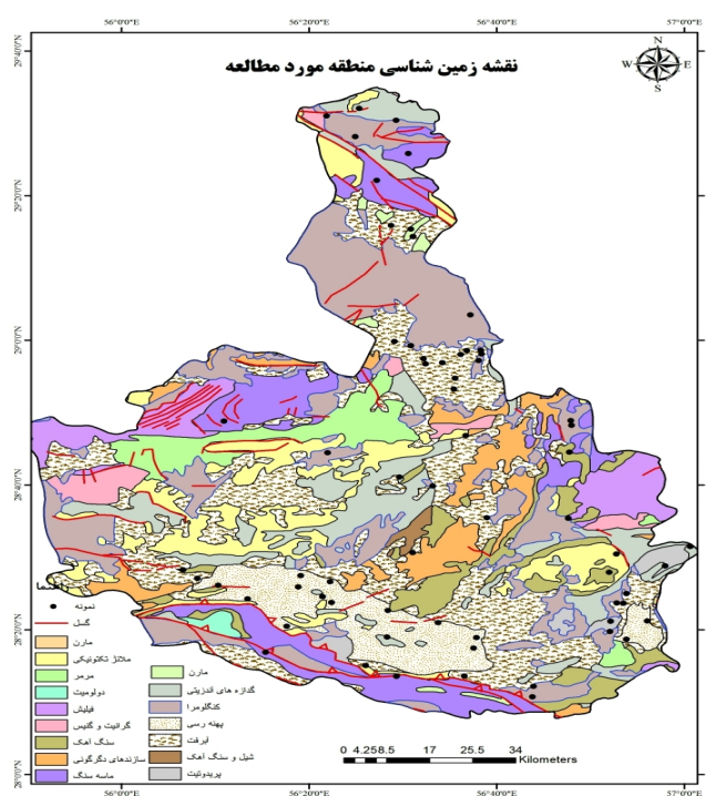
شکل ۲: نقشه زمین‌شناسی و گسلش منطقه مطالعه‌شده
