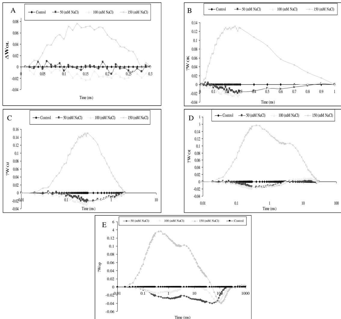
شکل ۱- بررسی تأثیر غلظت‌های متفاوت شوری بر میزان تغییرات فلورسانس نسبی کلروفیل a در گیاه جو دوسر در حواسط مراحل مختلف نمودار کینتیک فلورسانس کلروفیل a: (A) مرحله OL، (B) مرحله OK، (C) مرحله OJ، (D) مرحله OI، (E) مرحله OP
