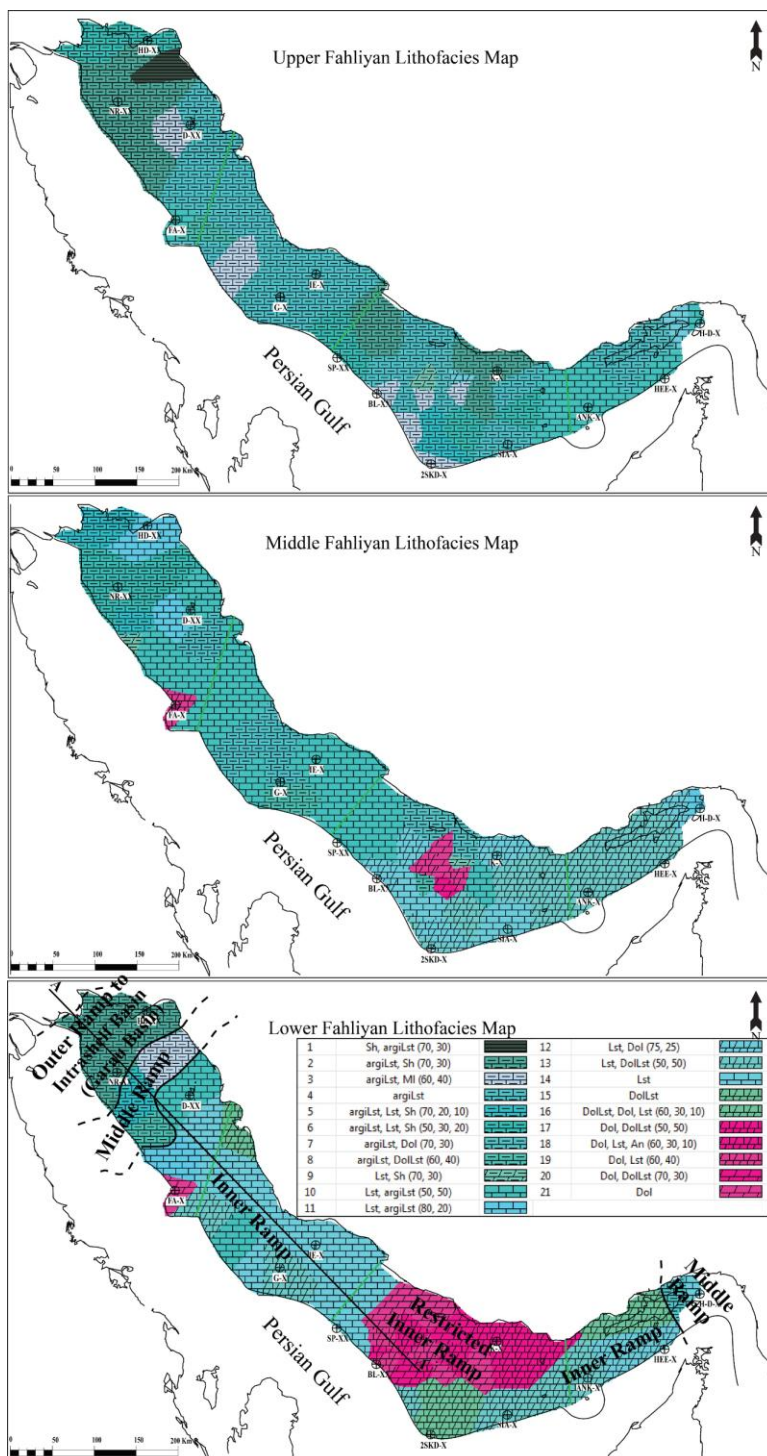
شکل ۱۲- نقشه توزیع رخساره‌های سنگی در بخش پایینی، میانی و بالایی سازند فهلیمان در خلیج فارس. زیر محیط‌های پلتفرم کربناته در بخش چینه‌شناسی پایینی مشخص گردیده است. ترانسکت A-A' در بخش پایینی سازند فهلیمان مربوط به شکل شماره ۱۱ است. رخساره سنگ آهک آرژیلیتی در بلوک B و C از گسترش قابل توجهی برخوردار است. رخساره‌های سنگی مربوط به حوضه عمیق بین پلتفرمی نیز که در بخش پایینی در بلوک D در اثر فعالیت گسل‌های پی سنگی وجود داشته است در این مرحله توسط رسوبات پلتفرم پر گردیده است و شواهدی از زبانه‌های سازند گرو در بخش میانی سازند فهلیمان وجود ندارد.
