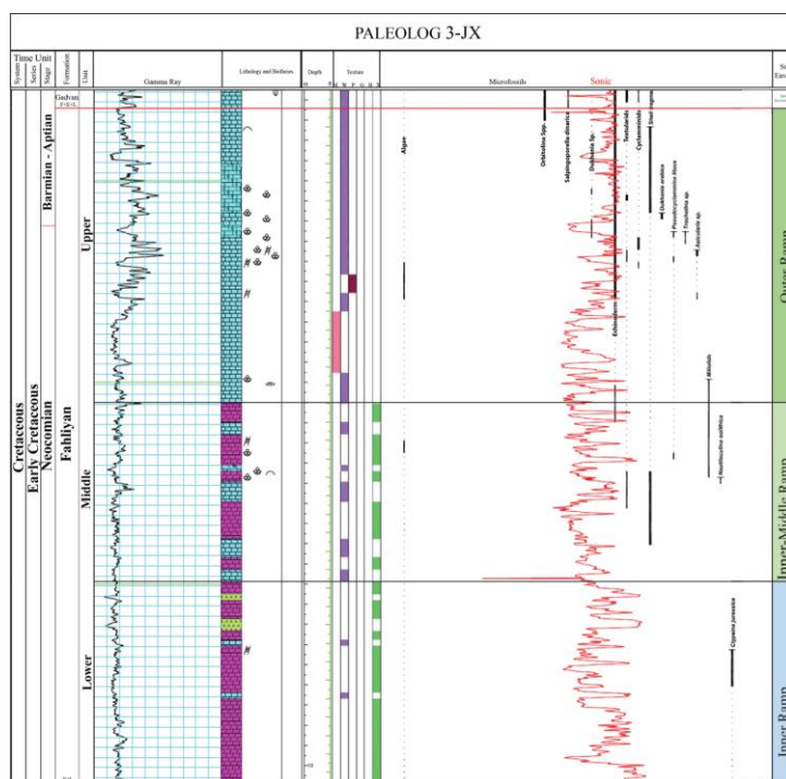
شکل ۶- ستون چینه‌شناسی سازند فهلیان در چاه 3J-X از ساختمان جاودان (اقتباس با تغییراتی از (Kalantari 2010)). برای مشاهده راهنما به شکل ۵ مراجعه نمایید.
