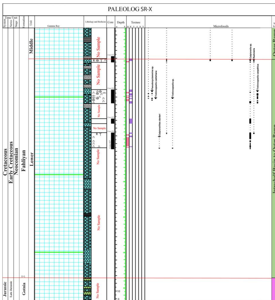
شکل ۹- ستون چینه‌شناسی بخش پایینی تا میانی سازند فهلیان در چاه SR-X از میدان سروش (اقتباس با تغییراتی از (Moghaddasi 2006)). برای مشاهده راهنما به شکل ۵ مراجعه نمایید.
