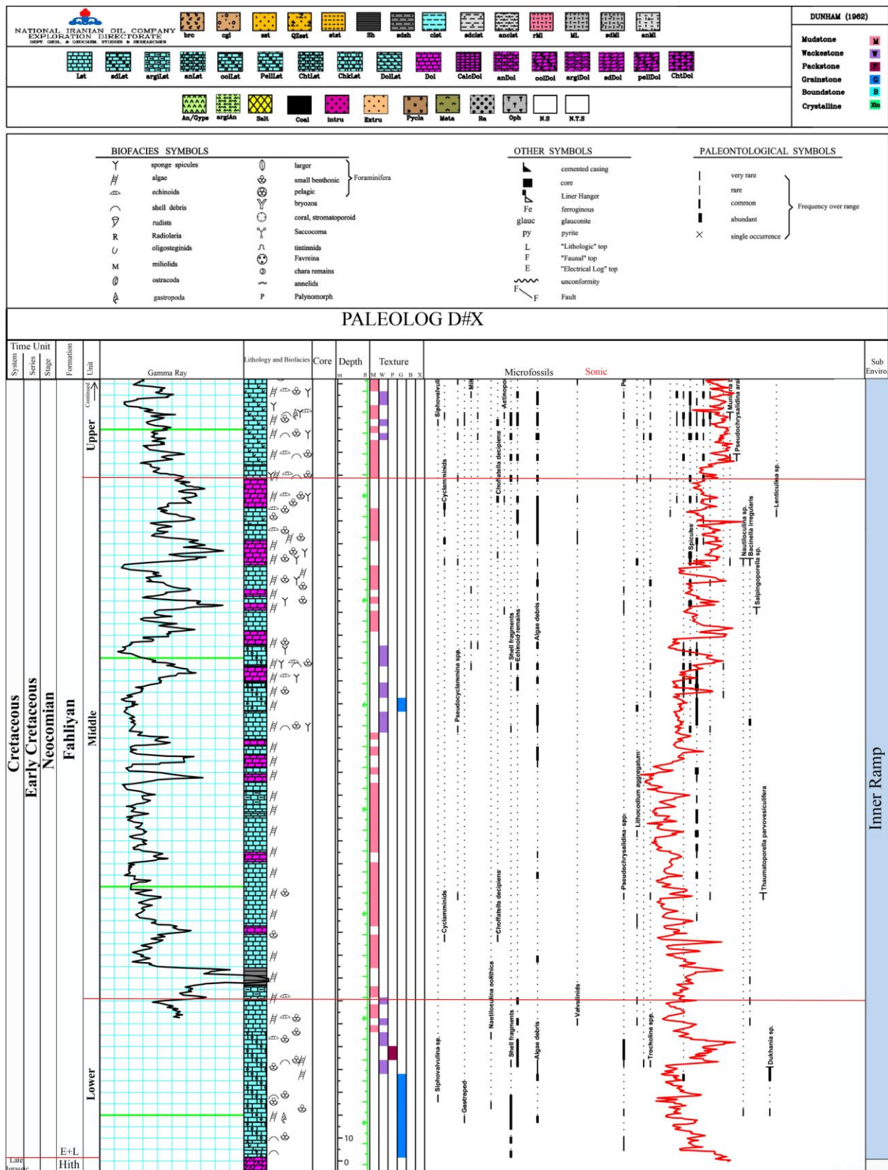
شکل ۵- ستون چینه‌شناسی بخش پایینی، میانی و ابتدای بخش بالایی سازند فهلایان در چاه D-X از میدان درود (اقتباس با تغییراتی از ( Mohammad Beigi 2007)). علائم ارائه شده در رهنمای بالای تصویر مربوط به شکل‌های ۹-۶ نیز است.
