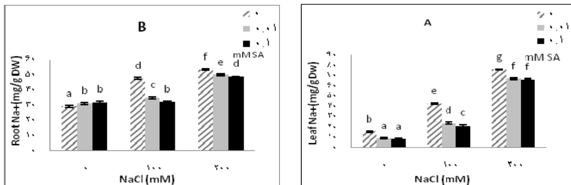
شکل ۳- اثر متقابل سالیسیلیک اسید و تنش شوری بر مقدار سدیم برگ (A) و ریشه (B). مقادیر، میانگین ۳ تکرار و مقایسه میانگین‌ها بر اساس آزمون LSD است. حروف یکسان بیانگر عدم اختلاف معنی‌دار در سطح P \leq 0.05 است.
