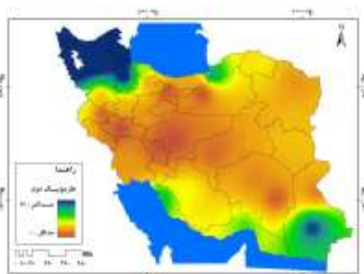
شکل ۶- درصد واریانس هارمونیک دوم (PVR2).
