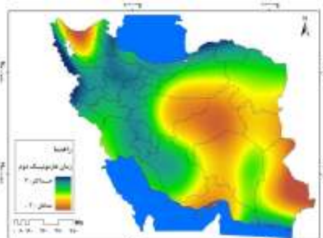
شکل ۷- زمان وقوع حداکثر مولفه هارمونیک دوم (TK2)
