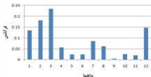
شکل ۳- فرکانس نسبی بارش ماهانه ایستگاه ایرانشهر
