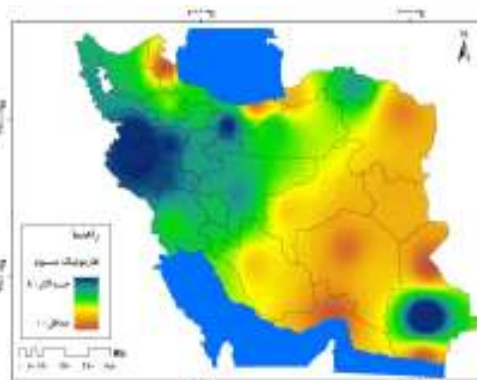
شکل ۸- درصد واریانس هارمونیک سوم (PVR3).
