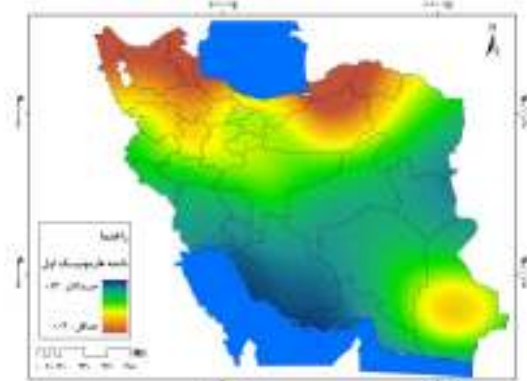
شکل ۱۰- دامنه هارمونیک اول (Ck1).
