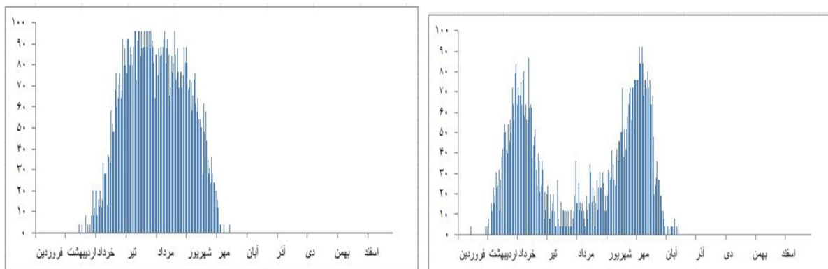
شکل ۷) درصد فراوانی ماهانه گونه‌هواهای گرم و نسبتاً شرجی (گونه ۵) شکل ۸) درصد فراوانی ماهانه گونه‌هواهای گرم و مرطوب شرجی (گونه ۶)
