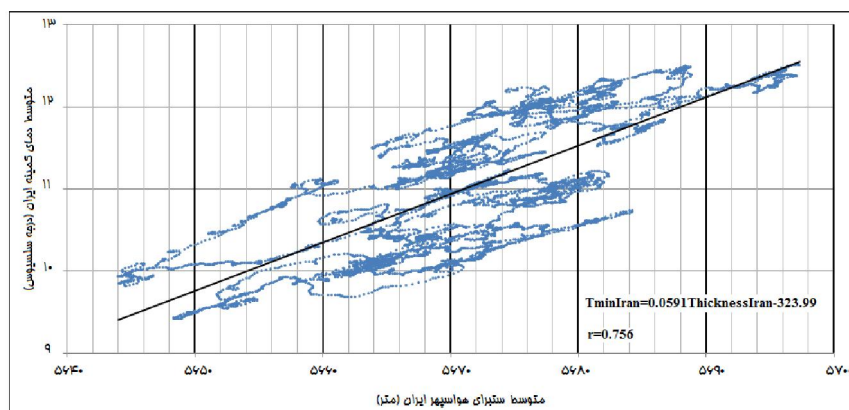
شکل ۶) همبستگی بین میانگین ستبرای هواسپهر ایران و میانگین دمای کمینه ایران
