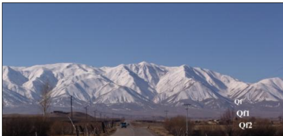
شکل ۸) نمایی از مخروط افکنه‌های بهم پیوسته دامنه شمالی رشته کوه بزقوش مخروط افکنه جوان = Qf مخروط افکنه جدید = Qf1 مخروط افکنه قدیمی = Qf2
