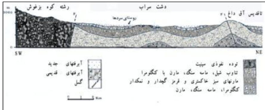
شکل ۴) مقطع زمین شناسی دامنه شمالی رشته کوه بزقوش (با تغییراتی از سازمان زمین شناسی، ۱۹۹۳)
