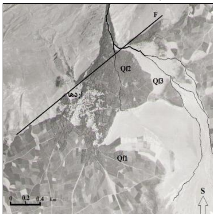
شکل ۹) عکس هوایی مخروط افکنه اردها در محل قطع شدگی آن با گسل شرق بزقوش مخروط افکنه پیشین = Qf1 مخروط افکنه پسین = Qf2 بخش فعال کنونی = F = گسل
