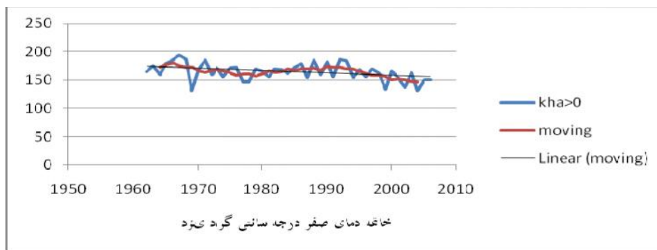
شکل ۱۱) تغییرات میانگین تاریخ خاتمه دمای صفر سانتیگراد در ایستگاه یزد
