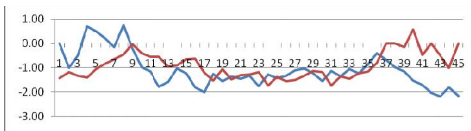
شکل ۸) نمودار u و u' تاریخ خاتمه دمای ۵ درجه سانتیگراد در ایستگاه یزد
