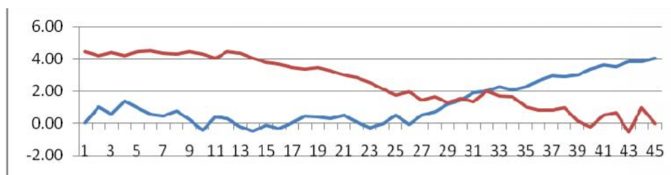
شکل ۶) نمودار ۵ و ۱۱ تاریخ آغاز دمای ۵ درجه سانتیگراد در ایستگاه یزد
