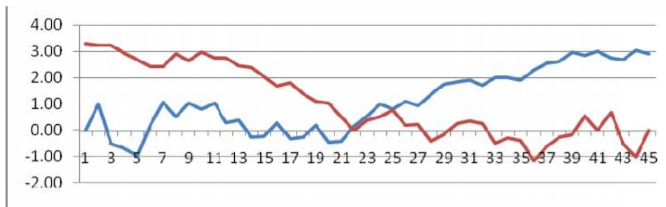
شکل ۱۰) نمودار \mu و \sigma تاریخ آغاز دمای صفر سانتیگراد در ایستگاه یزد
