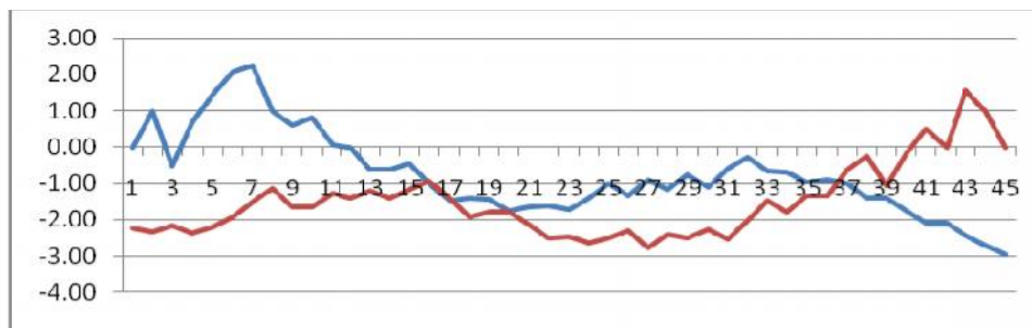
شکل ۱۲) نمودار \mu و \sigma تاریخ خاتمه دمای صفر سانتیگراد در ایستگاه یزد
