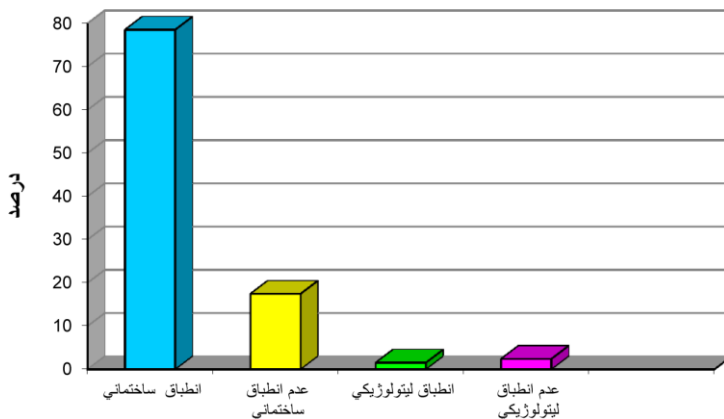
شکل (۴) درصد شبکه‌های انطباق یافته و انطباق نیافته ساختمانی، لیتولوژیکی، و گسلی
