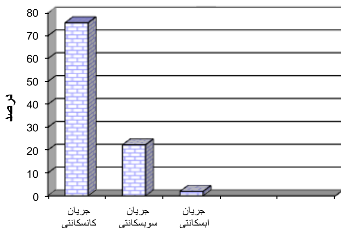
شکل (۳): درصد انطباق و عدم انطباق لیتولوژیکی شبکه‌های هیدروگرافی
