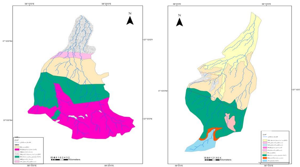
شکل (۹) شبکه‌های انطباق یافته و انطباق نیافته حوضه‌های سه گنبد و شیرغان
