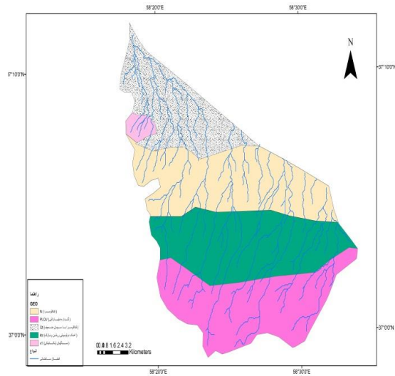
شکل (۷) شبکه‌های انطباق یافته و انطباق نیافته حوضه‌های مایوان و چری
