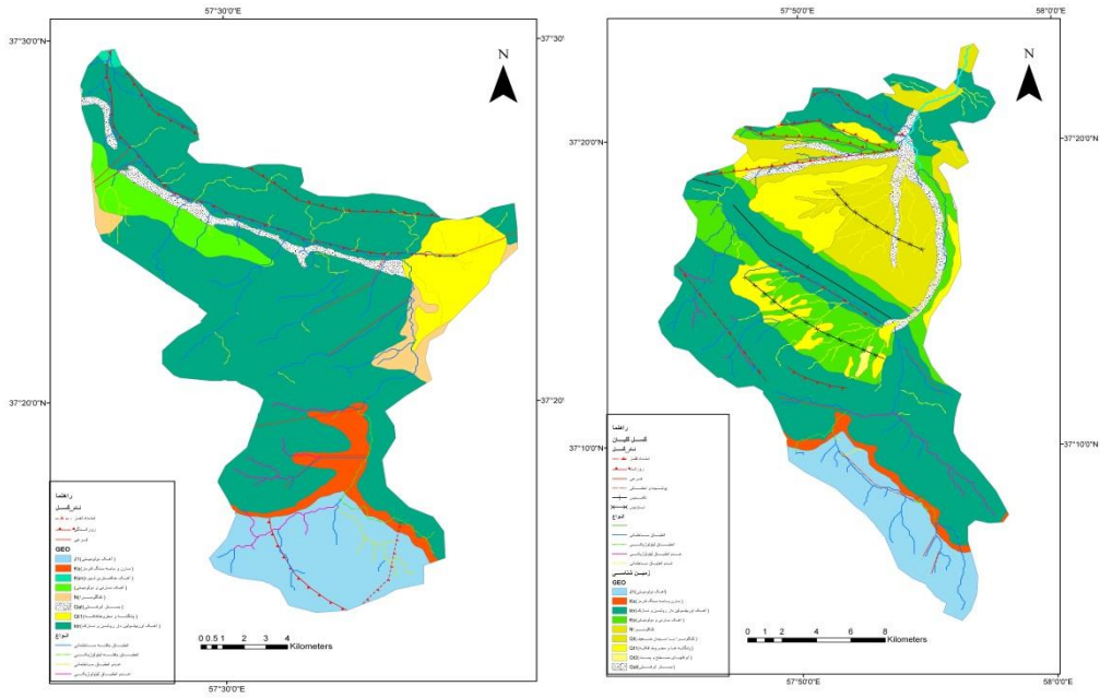
شکل (۵) شبکه‌های انطباق یافته و نیافته حوضه گلیان و اسفیدان
