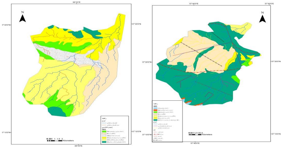
شکل (۶) شبکه‌های انطباق یافته و انطباق نیافته حوضه‌های زوارم و دوین
