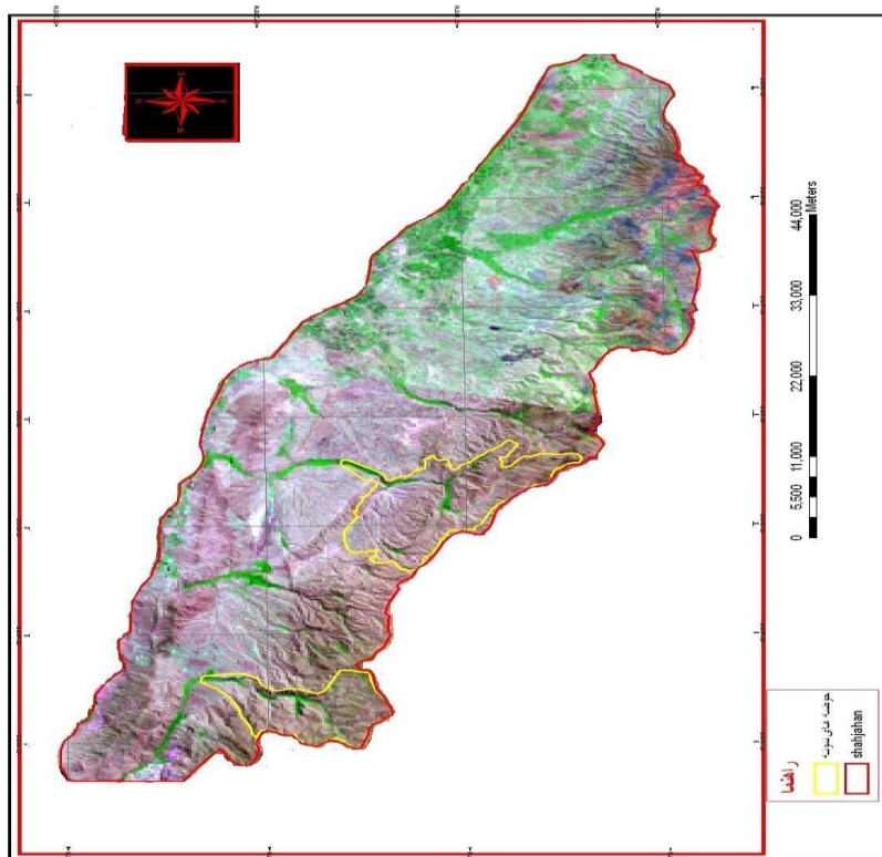
شکل (۱) موقعیت منطقه مورد مطالعه و موقعیت جغرافیایی دامنه‌های شمالی شاه جهان
