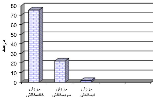
شکل (۲) درصد انطباق و عدم انطباق ساختمانی شبکه‌های هیدرولوژی
