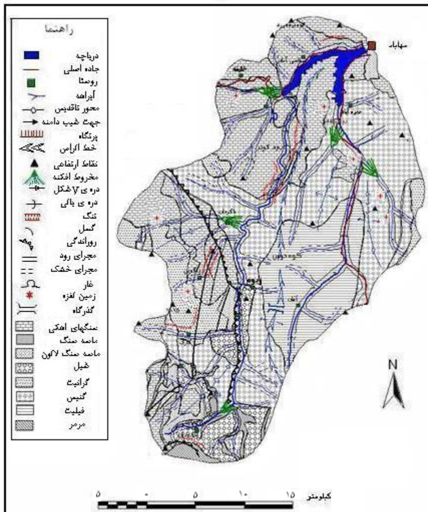
شکل ۲ نقشه زمین ریخت شناسی حوضه سد مهاباد
