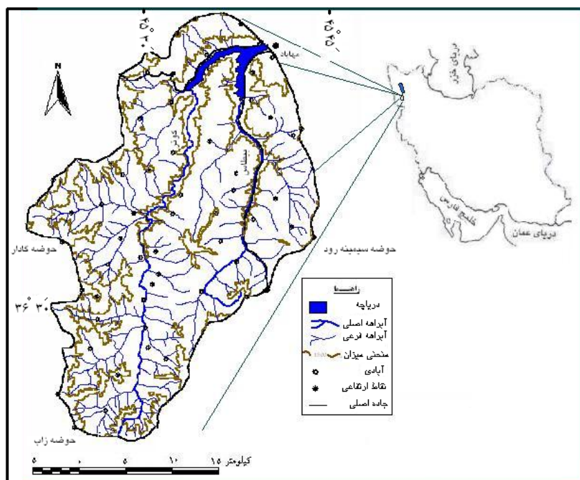
شکل ۱ موقعیت و وضعیت اوروهمیروگرافی منطقه مورد بررسی (حوضه بالادست سد مهاباد)
