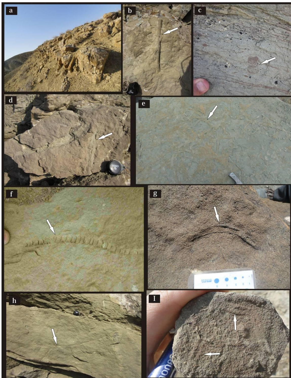
شکل ۴ (رخساره ۲): a: تناوب ماسه‌سنگ و افق‌های زیستی چگال، b: Ophiomorpha ، c: Teichichnus ، d: Rosselia socialis در برش قائم، e: Thalassinoides ، f: Taenidium ، g: Palaeophycus ، h: Cylindrichnus ، i: Gyrochorte
