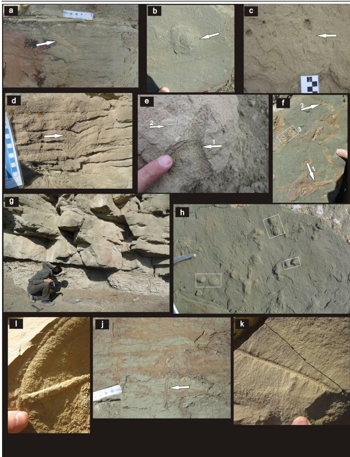
شکل ۸ - (رخساره ۴) - a: Cylindrichnus , b: Monocraterion? , c: Macaronichnus , d: Conichnus , e: O. nodosa (1) و Macaronichnus (2), f: Rosselia (1), O. nodosa (2), Arenicolites (3), g: ایکنوفاسیس، h: Thalassinoides با Diplocraterion ، i: O. irregular ، j: O. nodosa ، k: Skolithos
