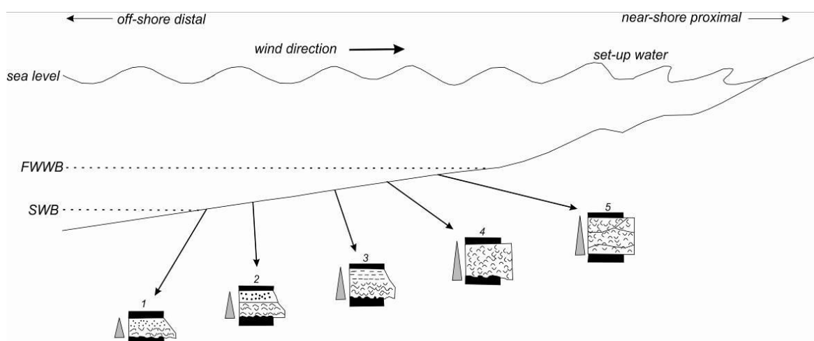
شکل ۱۱- روند پروکسیمال-دیستال افقهای پرفسیل در برش مورد مطالعه (FWWB: fair-weather wave base) موجسار هوای آرام، SWB: storm weather wave base موجسار هوای طوفانی).
