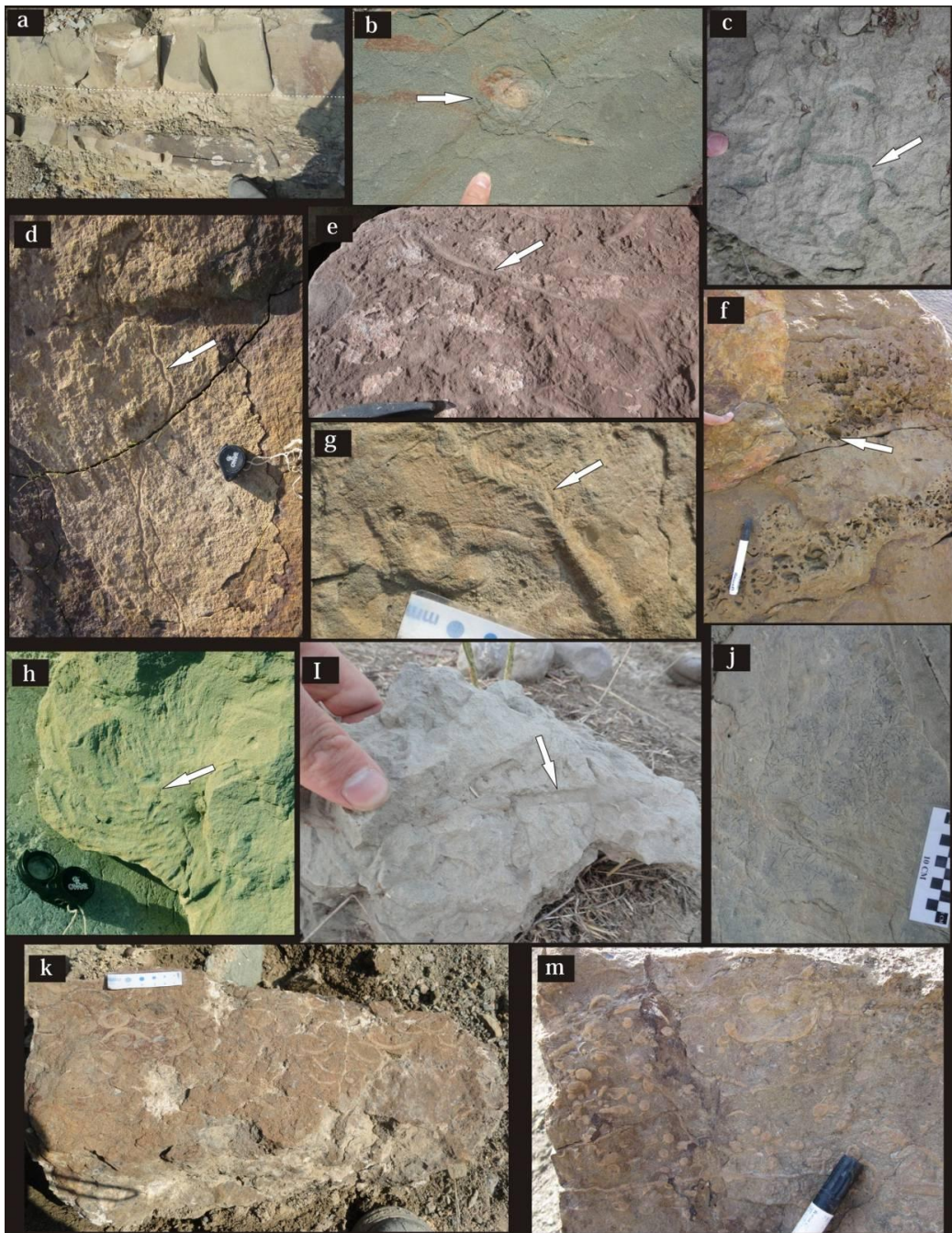
شکل ۳ (رخساره ۱) - a: لایه های ماسه سنگی به طور غالب به صورت توده ای با سطح قاعده فرسایشی، b: Rosselia ، c: Helminthopsis ، d: Gordia ، e: Planolites ، f: Gastrochaenolites همراه با قالب های صدف و افق های پرفسیل، g: Protovirgularia ، h: Zoophycos ، i: مادستون با زیست آشفستگی بالا شامل Ophiomorpha ، j: Chondrites و k و m: افق های پرفسیل
