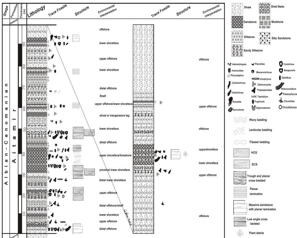
شکل ۲- ستون چینه شناسی سازند آیتامیر در برش امیرآباد
