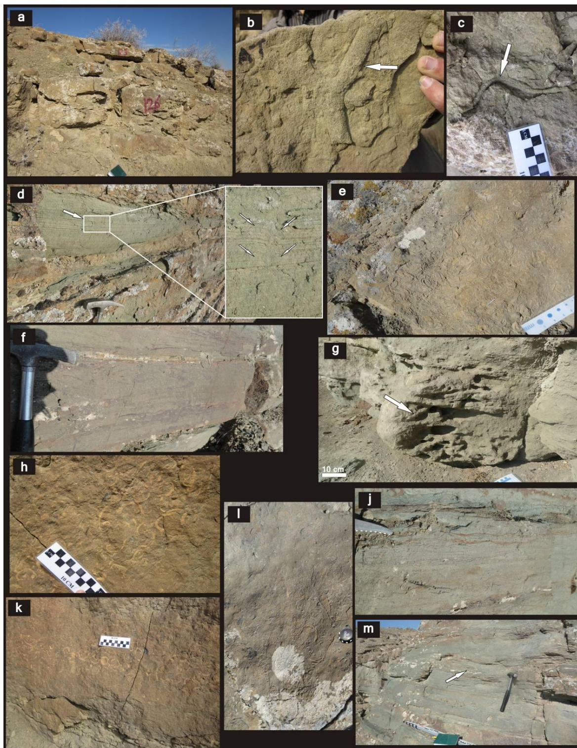
شکل ۶ (رخساره ۳)- a: توالی افق زیستی چگال و ماسه‌سنگ در بخش پایینی حاشیه ساحلی، b: Thalassinoides ، c: افق زیستی چگال با Ophiomorpha ، d: طبقه‌بندی مورب پشته‌ای با ساختارهای فراری در وسط، e: افق‌های پرفسیل، f: ساختارهای پیچ‌وتاب خورده ( navichnia )، g: Thalassinoides ، h و i: افق‌های پرفسیل، j: لامیناسیون ریپلی موجی و جریانی، k: افق‌های پرفسیل m: طبقه‌بندی مورب تقعر
