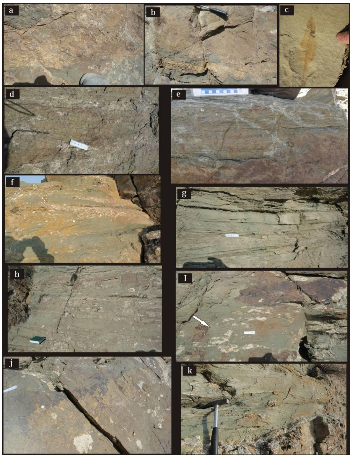
شکل ۷ (رخساره‌ها) - a و b: افق‌های پرفسیل، c: آثار برگ d: طبقه‌بندی مورب تابلار به سمت بالا به طبقه‌بندی مورب پشته‌ای، e: لامیناسیون ریپلی جریانی و ساختارهای فراری، f: طبقه‌بندی مورب پشته‌ای بزرگ مقیاس، g: طبقه‌بندی مورب تابلار با زاویه کم، h: طبقه‌بندی مسطح و کم زاویه، i: طبقه‌بندی مورب تراف، j: افق‌های پرفسیل، k: طبقه‌بندی مورب تراف در جهات مختلف بر روی هم
