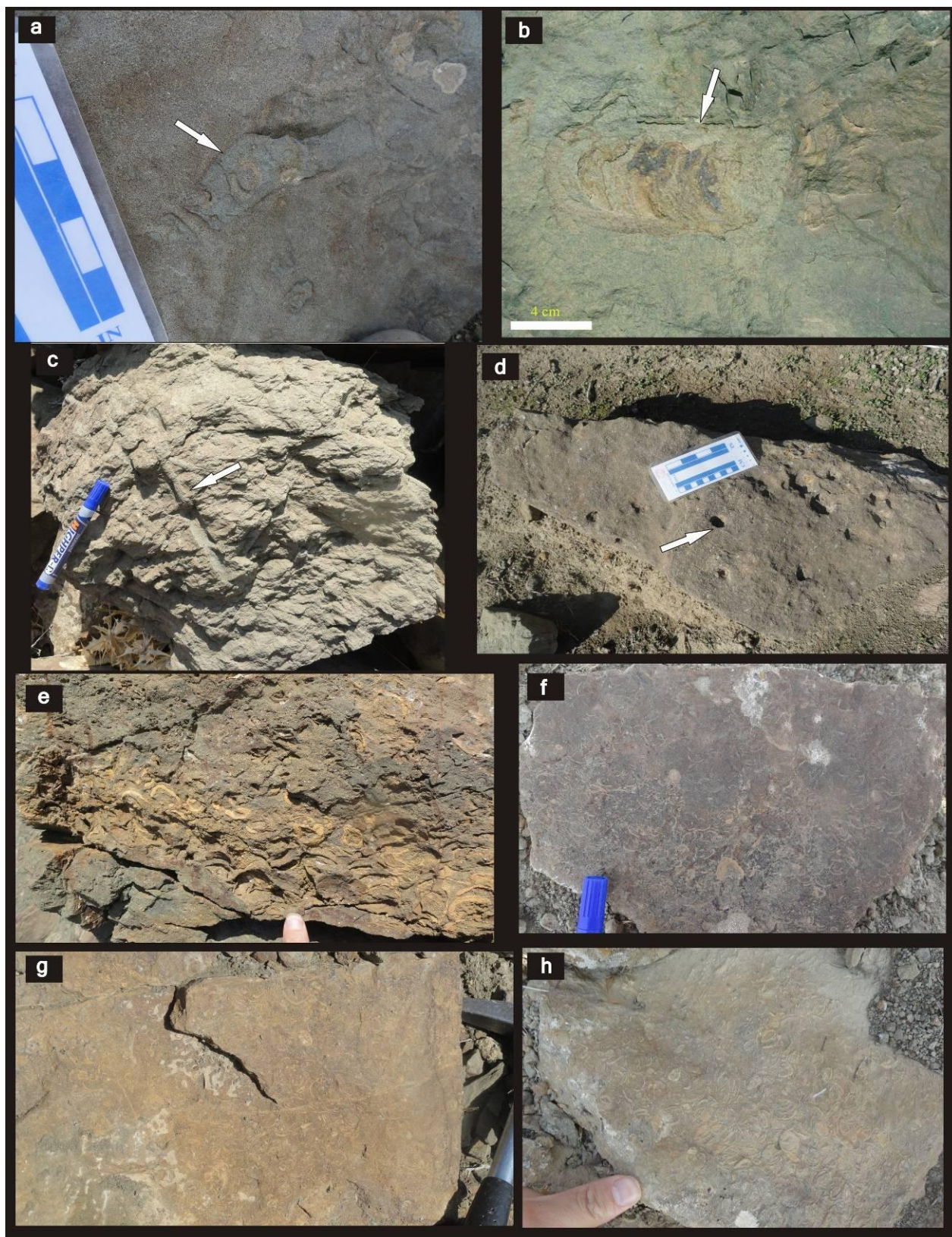
شکل ۵ (رخساره ۲) - a: Rhizocorallium , b: Rosselia socialis , c: مادستون با زیست آشفته‌گی بالا حاوی O. nodosa و Thalassinoides , d: Gastrochaenolites , e تا h: افق‌های پرفسیل
