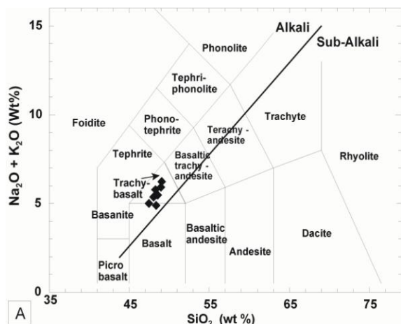
شکل ۶- نامگذاری سنگ‌های ولکانیک کوه توپره، (A) در نمودار \text{Total Alkalis}-\text{SiO}_2 ، TAS (Le Maitre, 2002) و (B) نمودار \text{Zr}/\text{TiO}_2\text{-Nb}/\text{Y} (Winchester and Floyd, 1977).
