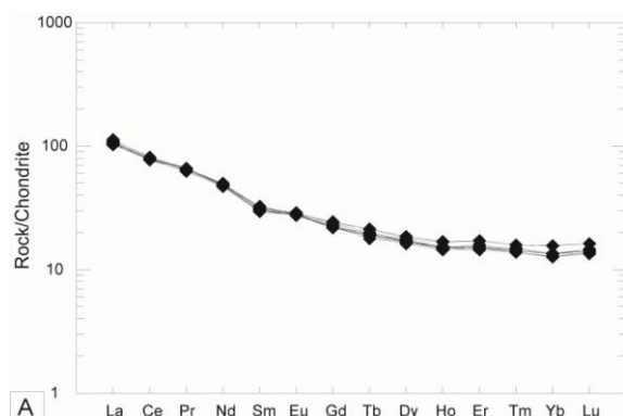
شکل ۷- نمودار بهنجار شده به کندریت (A) و (B) گوشته اولیه بازالت آلکالن توپره. داده‌های کندریت (Mc Donough and Sun, 1995) و داده‌های گوشته اولیه (Sun and Mc Donough, 1989).
