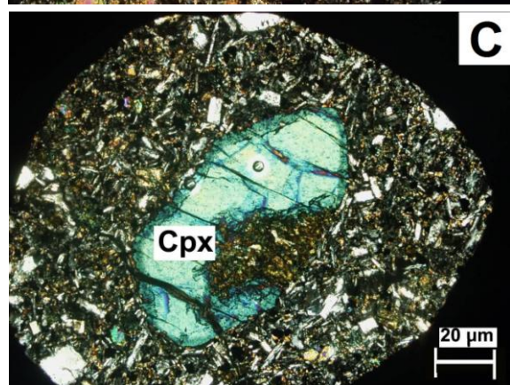
شکل ۴- تصاویر میکروسکوپی از بازالت آکالن تویره، همه تصاویر در نور پلاریزه است.
