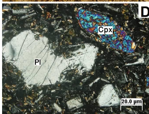
شکل ۴- تصاویر میکروسکوپی از بازالت آکالن تویره، همه تصاویر در نور پلاریزه است.
