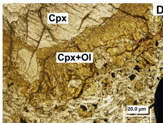
شکل ۵- تصاویر میکروسکوپی از زنوکریست‌ها و بافت‌های واکنشی آنها در بازالت آلکالن تویره، تصاویر A، B و C در نور پلاریزه و تصویر D در نور طبیعی است.
