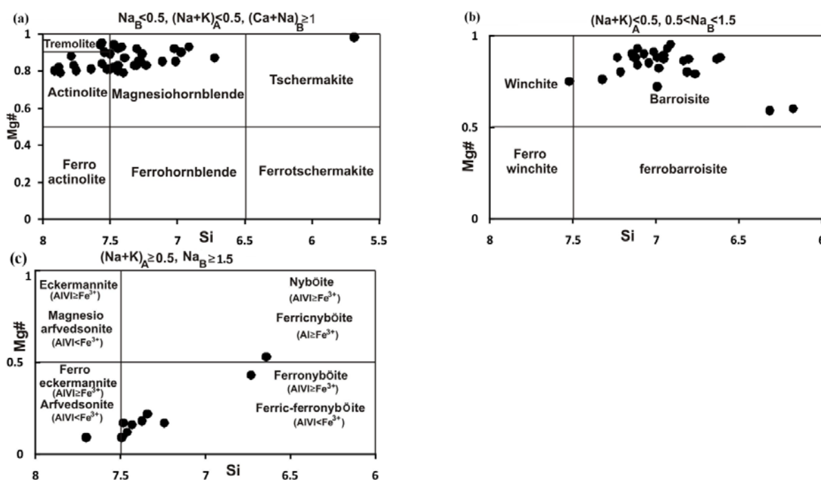
شکل ۹- مطابق پارامترها و نمودارهای تقسیم‌بندی آمفیبول‌ها (Leake et al. , 2004) آمفیبول‌های مورد مطالعه اغلب از نوع: (a) منیزیوهورنبلند و اکتینولیت، (b) باروینزیت، و (c) فریک‌فرونیبوئیت و آرفودسونیت \{AIVI < Fe^{3+}\} هستند.
