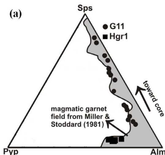
شکل ۱۳- با توجه به نمودار سه‌تایی متمایزکننده گارنت‌های ماگمایی از انواع دگرگونی (Miller and Stoddard, 1981) گارنت‌های مورد مطالعه در قلمرو گارنت‌های ماگمایی قرار می‌گیرند.
