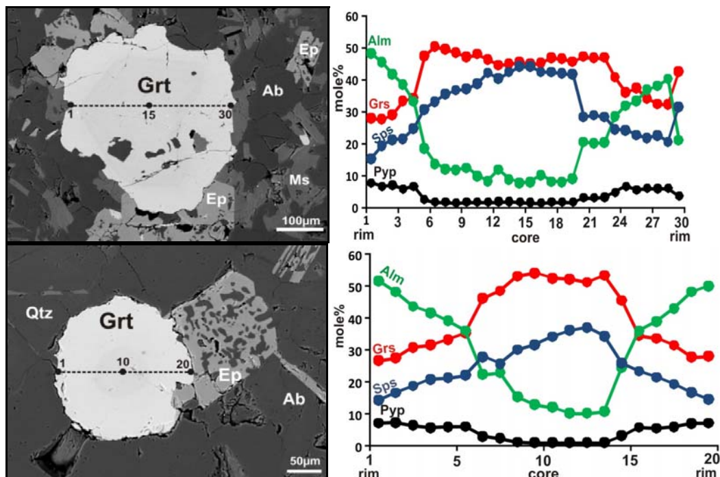
شکل ۱۱- تصاویر BSE دو عدد از گارنت‌های نمونه G11. این گارنت‌ها منطقه‌بندی ترکیبی بارزی را نشان می‌دهند. مقادیر سازنده‌های گروسولار و اسپسارتین از مرکز به طرف حاشیه کاهش و میزان آلماندین و پیروپ افزایش می‌یابد. کاهش متشکله گروسولار در حاشیه بیانگر تبلور گارنت در هنگام صعود ماگماست.
