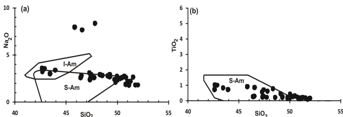
شکل ۱۰- در نمودارهای متمایز کننده آمفیبول ماگماهای داخل صفحه‌ای از انواع موجود در مناطق فرورانش (Coltorti et al., 2007) ترکیب شیمیایی آمفیبول‌های مورد مطالعه غالباً در محدوده آمفیبول‌های مناطق فرورانش قرار می‌گیرند (I-Am: آمفیبول ماگماهای داخل صفحه‌ای و S-Am: آمفیبول مناطق فرورانش).
