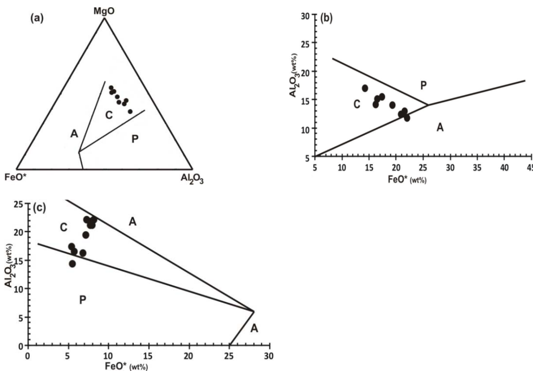
شکل ۱۵- در نمودارهای متمایزکننده محیط تکتونیکی با استفاده از ترکیب شیمیایی بیوتیت توده‌های ترونجمیتی منطقه از نوع ماگماهای کالک‌آلکان مناطق کوهزایی هستند (A: ماگماهای آلکان مناطق غیر کوهزایی، C: ماگماهای کالک‌آلکان مناطق کوهزایی (ماگماهای نوع I، P: ماگماهای پرآلومینوس (ماگماهای نوع S).
