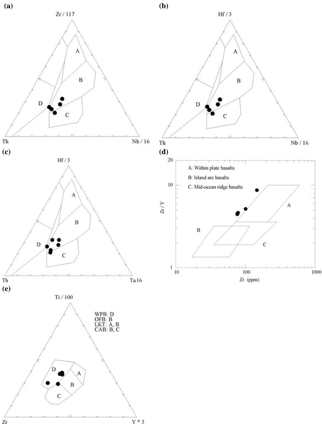
شکل ۹- نمودار تعیین موقعیت تکتونیکی بازالت‌های منطقه پل خاوند، (a) نمودار Zr/117 - Th - Nb/16 ، (b) نمودار Hf/3 - Th - Nb/16 ، (c) نمودار Hf/3 - Th - Ta (Wood, 1980) (محدوده A: مورب نوع N، محدوده B: مورب نوع E و بازالت‌های تولیتی درون صفحه‌ای، محدوده C: بازالت‌های درون صفحه‌ای و محدوده D: بازالت‌های قوس آتشفشانی)، (d) نمودار Zr/Y - Zr (Pearce and Norry, 1979) (B: بازالت‌های قوسی، C: مورب، A: بازالت‌های درون صفحه‌ای)، (e) تغییرات در محتوی نسبی Ti ، Zr و Y بازالت‌های مربوط به محیط‌های تکتونیکی مختلف (Pearce and Cann, 1973) (LKT: تولیت‌هایی با پتاسیم کم، CAB: بازالت‌های کالک‌آلکالن، OFB: بازالت‌های کف اقیانوسی، WPB: بازالت‌های درون قاره‌ای).
