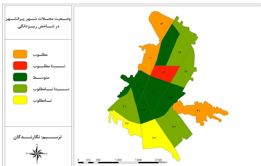
شکل ۷- آسیب‌پذیری شهر پیرانشهر در برابر زلزله با در نظر گرفتن شاخص ریزدانی
