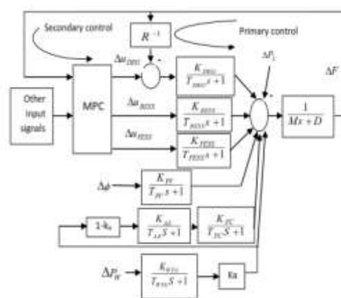
شکل (۲): مدل دینامیکی ریزشبهه
