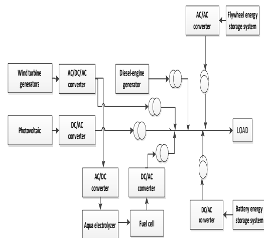
شکل (۱): شماتیک ریزشبکه [۳۶]
