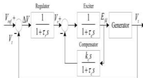
شکل (الف-۱): بلوک دیگرام سیستم تحریک دیزل ژنراتور
