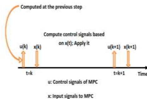
شکل (۴): ترتیب زمانی سیگنال‌ها در کنترل‌کننده پیش‌بین
